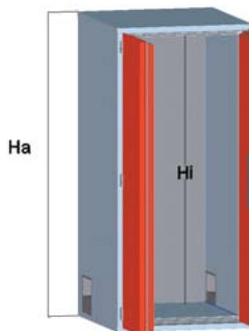
Модульный сейф высотой 47 HU (42 HU) с одной одинарной и одной двойной дверями
